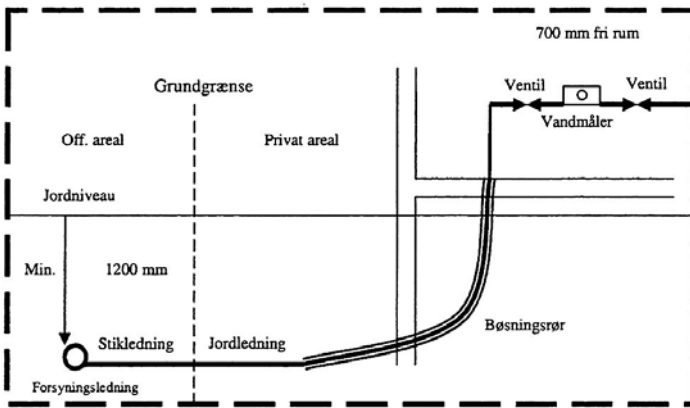
Figur 1: Vejledende eksempel på indføring af stik- og jordledning samt krav til vandmålerinstallation.
